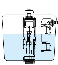
TORNEIRA DE BÓIA NA POSIÇÃO FECHADA
