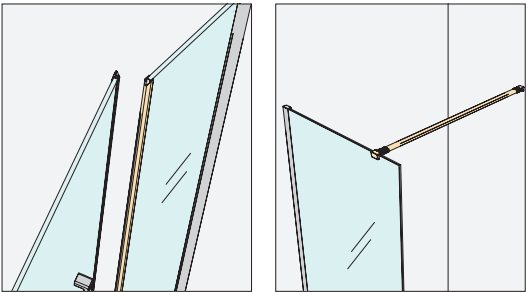
Kit fecho magnético
