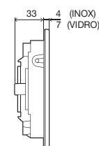
mecânico
