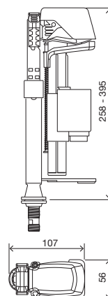
Aplicação inferior
