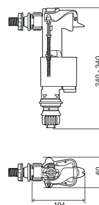
Aplicação lateral
