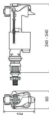
Aplicação inferior
