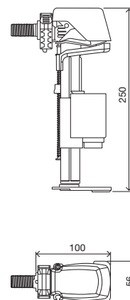
Aplicação lateral
