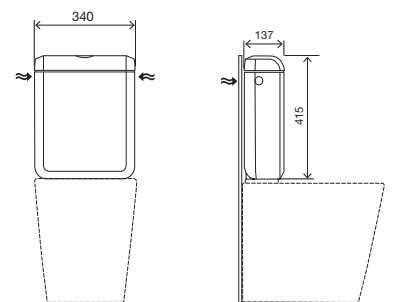
Aplicação monobloco
