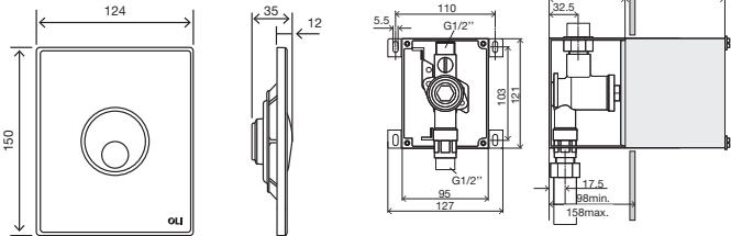
Caixa de pré-instalação do urinol
