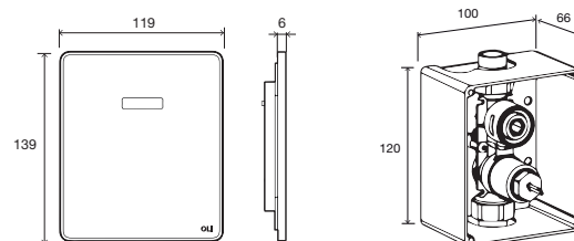
Caixa de pré-instalação do urinol
